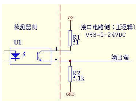
图 4：正逻辑接法
