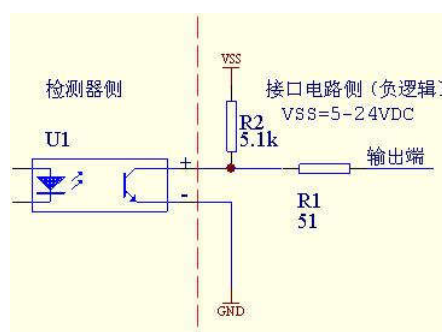
图 5：负逻辑接法
