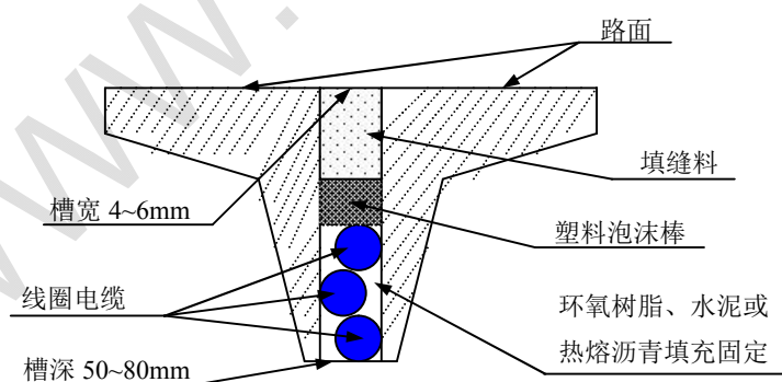
图 7：线槽截面示意图
