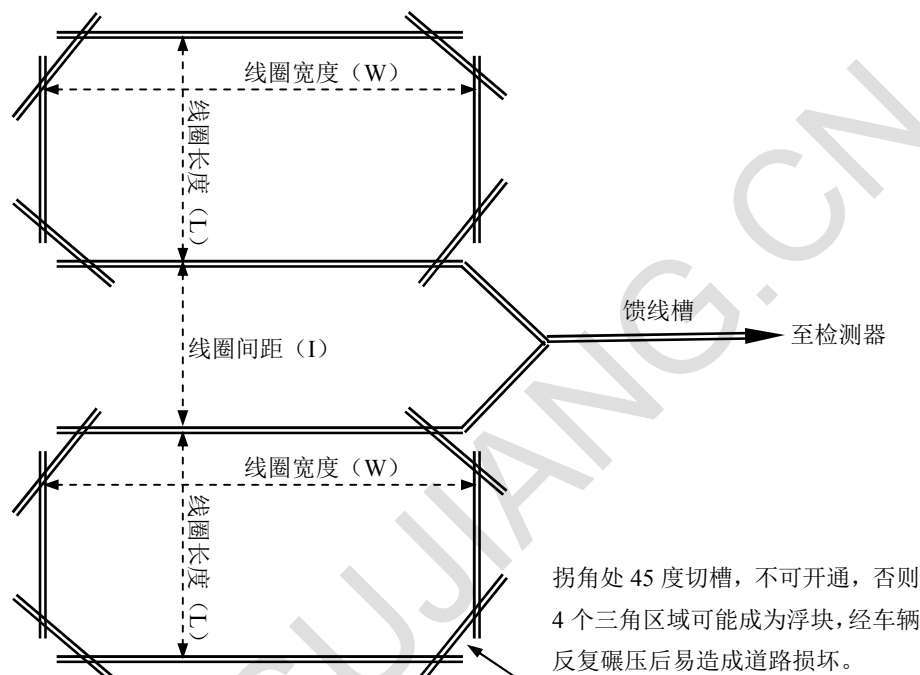
图 6：路面开槽示意图
