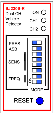
图 2：前面板
